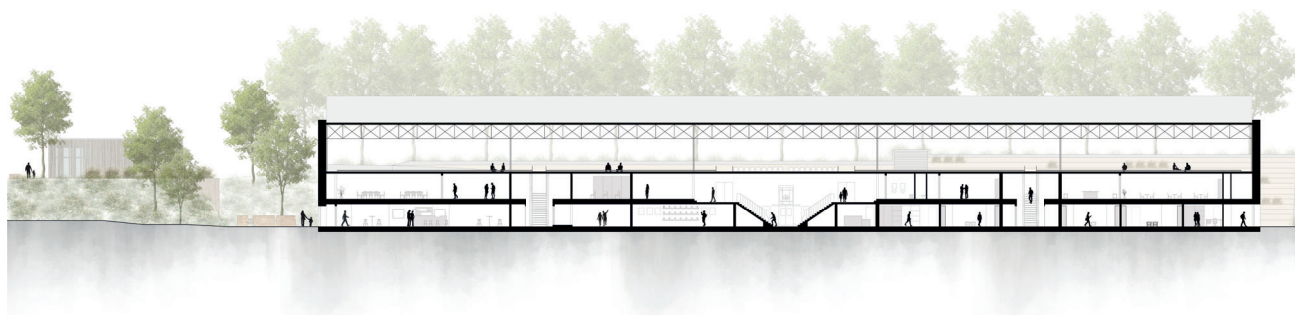
Coupe longitudinale du bâtiment historique
