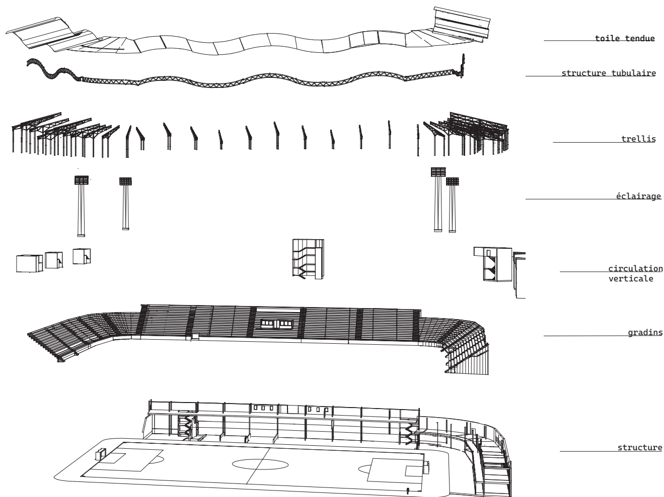
Schéma du principe structurel et éléments fonctionnels
