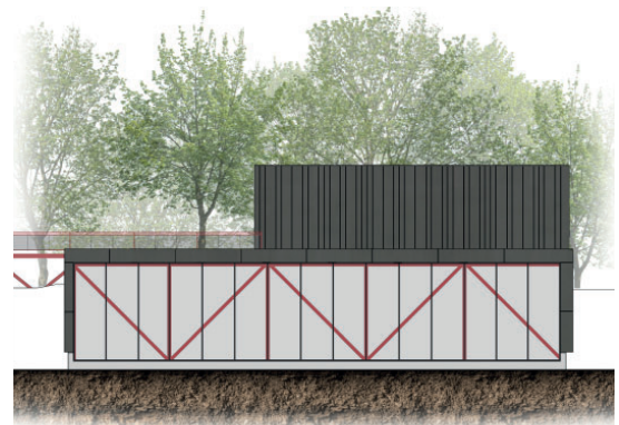
Façade nord B
